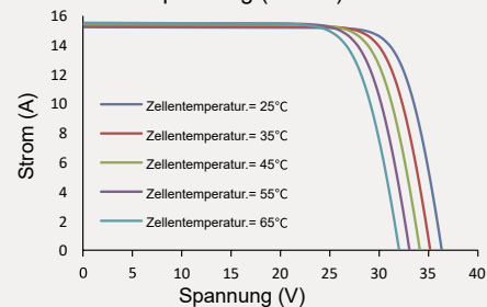
Strom-Spannung (445 W)
