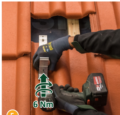
5 Die Stütze ( 6 \text{ Nm} \pm 0,5 \text{ Nm} ) fest verschrauben.
